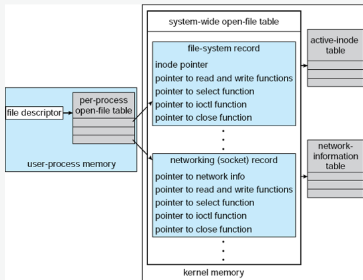
Figura 4. Estructuras de datos E/S en UNIX.
